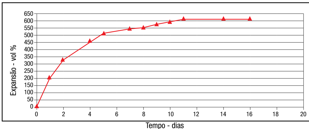
Fig. 1: gráfico de expansão do volume de Idrostop Soft em água destilada a +25°C de acordo com a norma JIS K6258:1993
